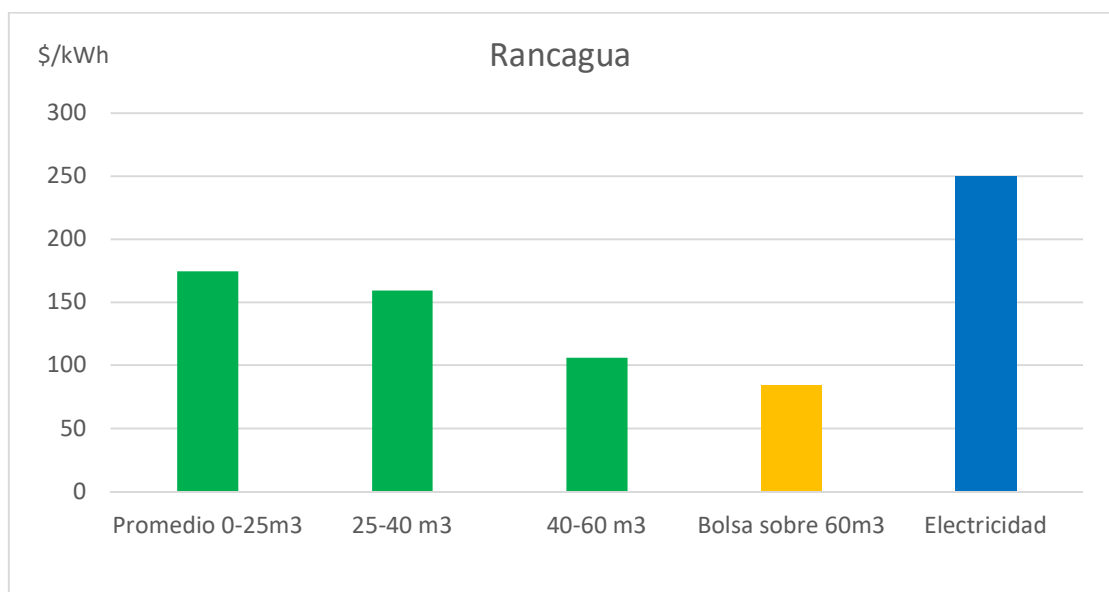
Figura 2: Costo por unidad de energía en Rancagua
