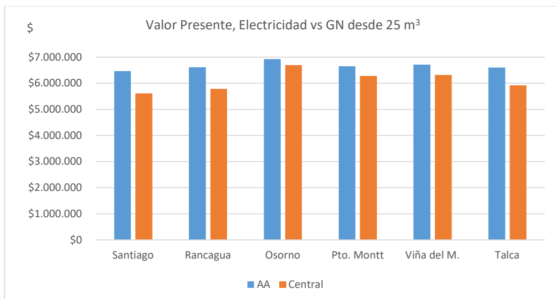
Figura 15: Valor presente considerando electricidad (inversión máxima) y un precio sobre 25 m 3 para el gas natural (inversión promedio).
