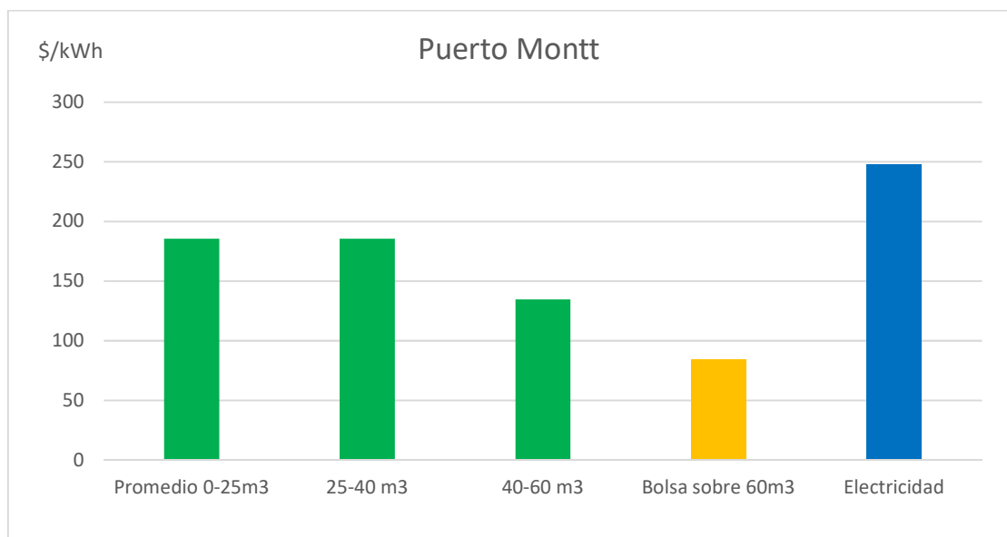
Figura 4: Costo por unidad de energía en Puerto Montt
